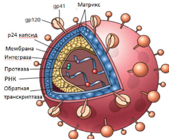
Рисунок 1. Структура ВИЧ.
