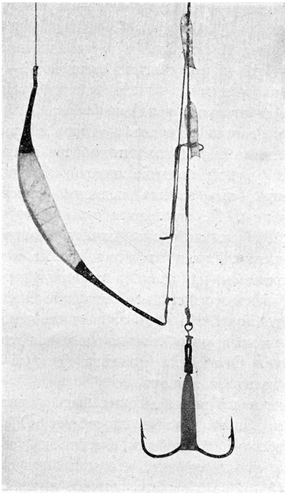
Снасть для лова на поддевъ. Внизу — крючки; вверх по лесе — металлическія рыбки для приманки; слева — грузило.
